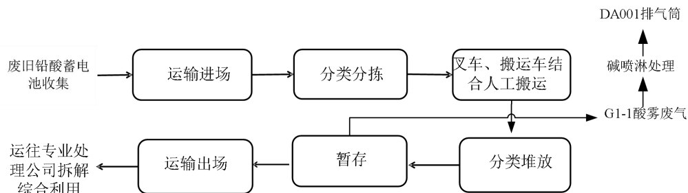
图 4-1 建设项目整体生产工艺流程及产污示意图
